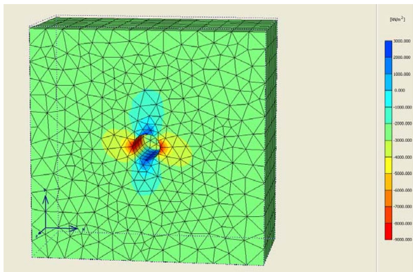
Рисунок 2 – Пример реализации метода конечных элементов
